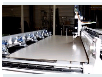
MACHINE DE DÉCOUPE
