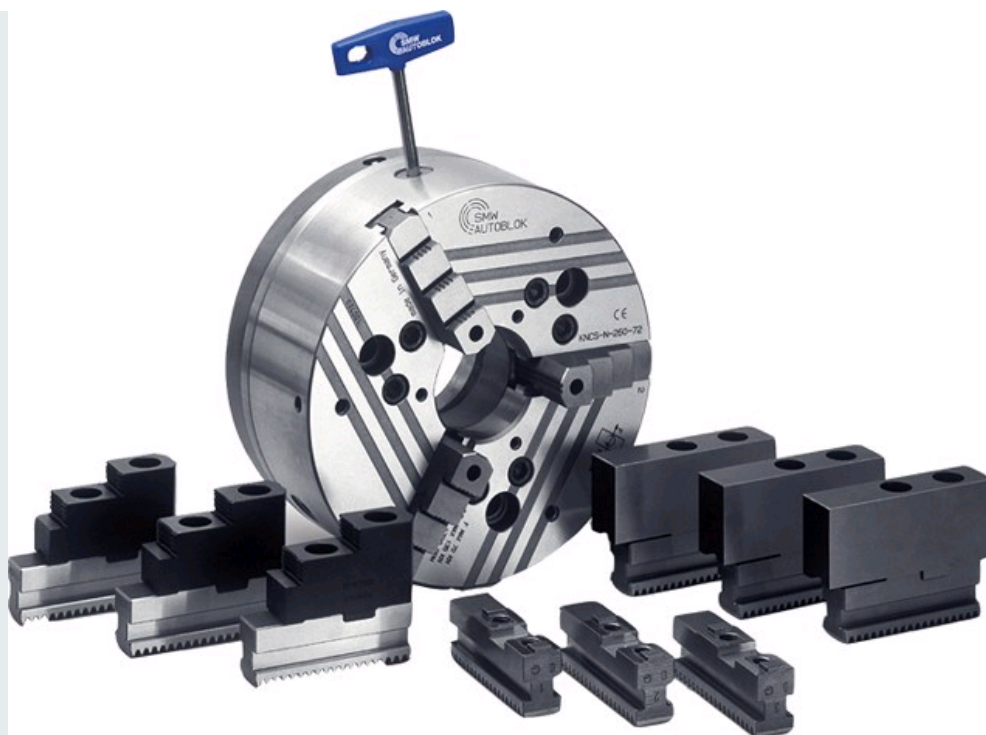
MANDRIN KNCS-N À CHANGEMENT RAPIDE DE MORS PAR CRÉMAILLÈRE
