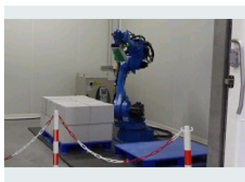
DÉMONSTRATION DE PALETTISATION
