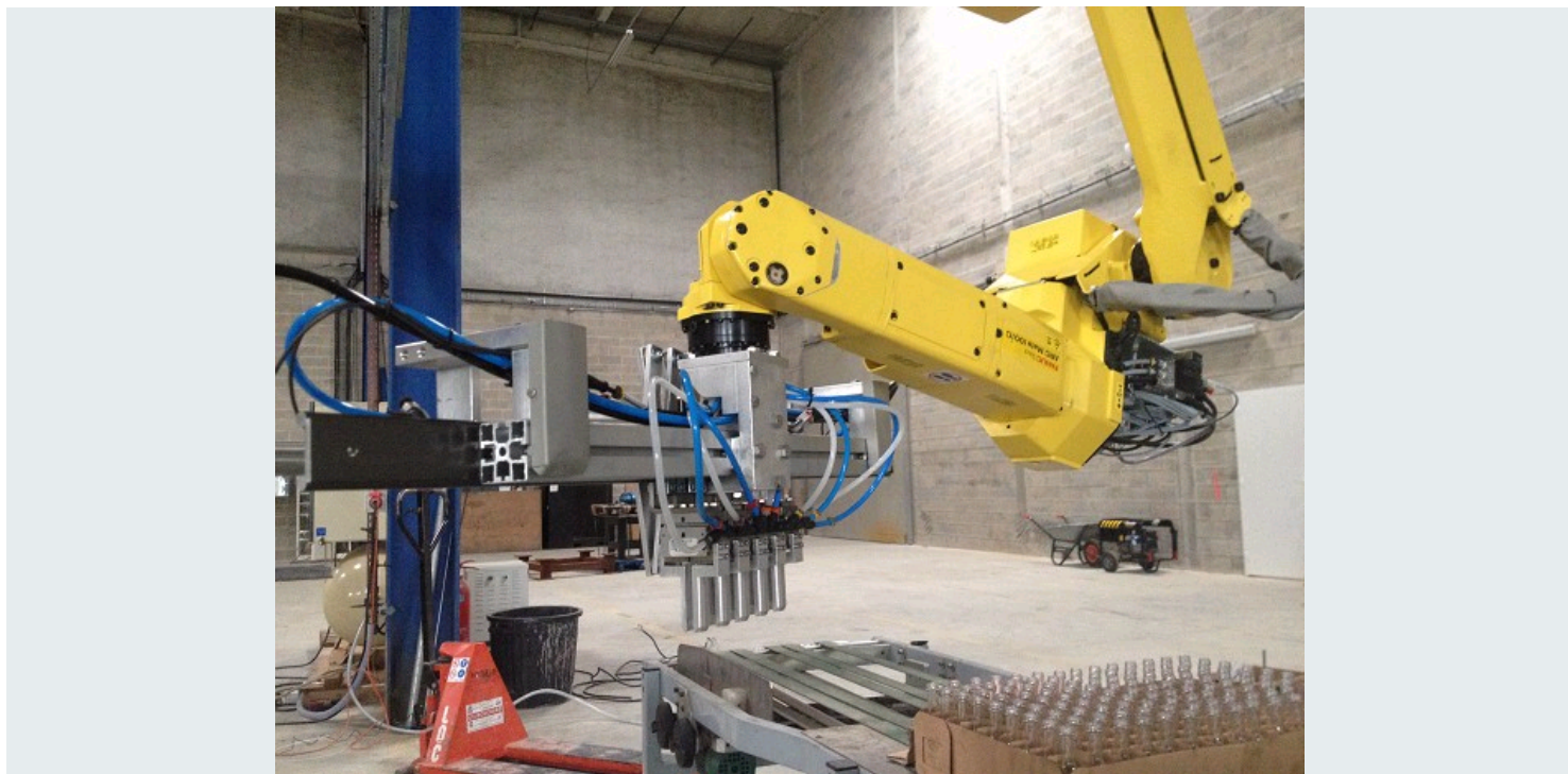
CHARGEMENT ET DECHARGEMENT DE BOUTEILLES POUR INDUSTRIE VERRIER
