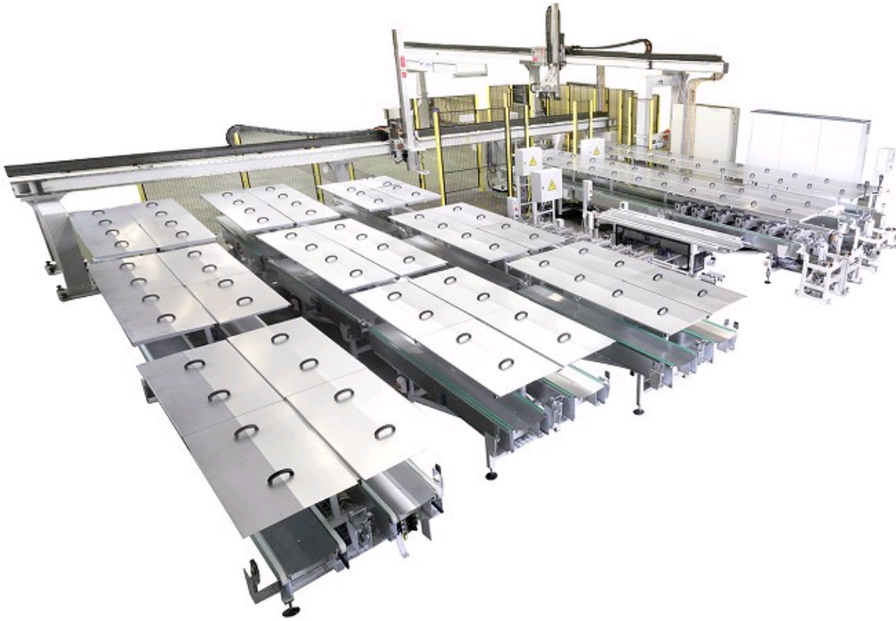
MANIPULATION ET STOCKAGE DE CULASSES MOTEUR ENTRE USINAGE ET ASSEMBLAGE
